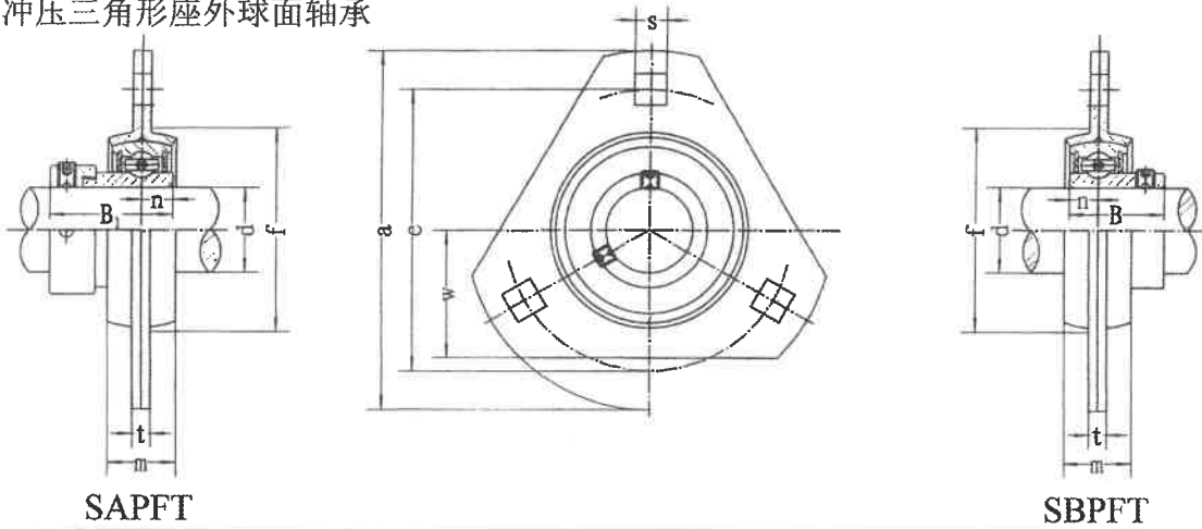
带冲压三角形座外球面轴承
